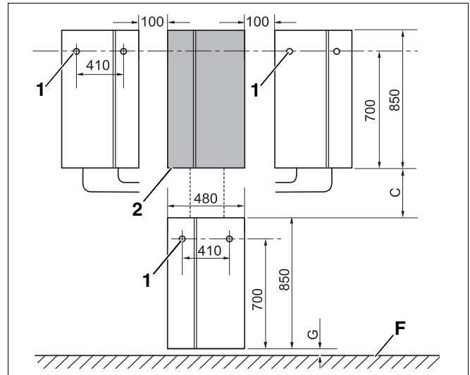
Sl. 4 Postavljanje (dimenzionalna skica)
