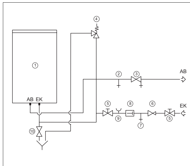
Sl. 9 Shema instalacije (principni prikaz)
