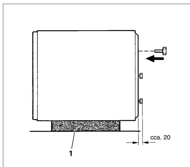
Sl. 3 Spremnik na jastuku poklopca (principna slika)
