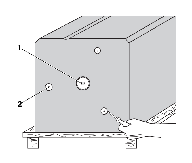
Sl. 5 Pogled odozdo: montaža kompleta za pražnjenje
