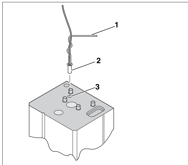
Sl. 10 Montaža senzora (principna skica)
