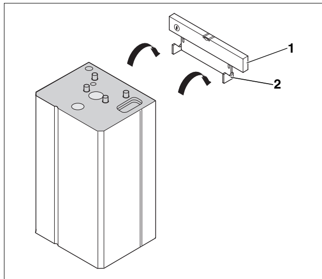
Sl. 6 Montaža vješanjem (priključak odozgo)
